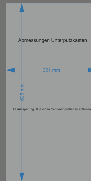
WANDAUSSPARUNG TSU 600 LONG
